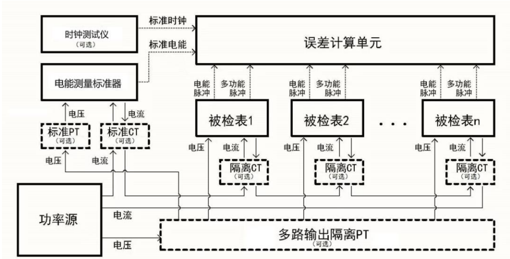
图 1 交流电能表检定装置典型线路原理框图
